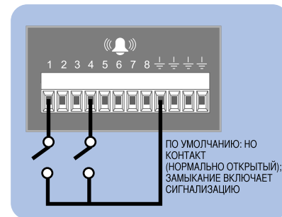
Рис. 5. Подсоединение сигнализации
